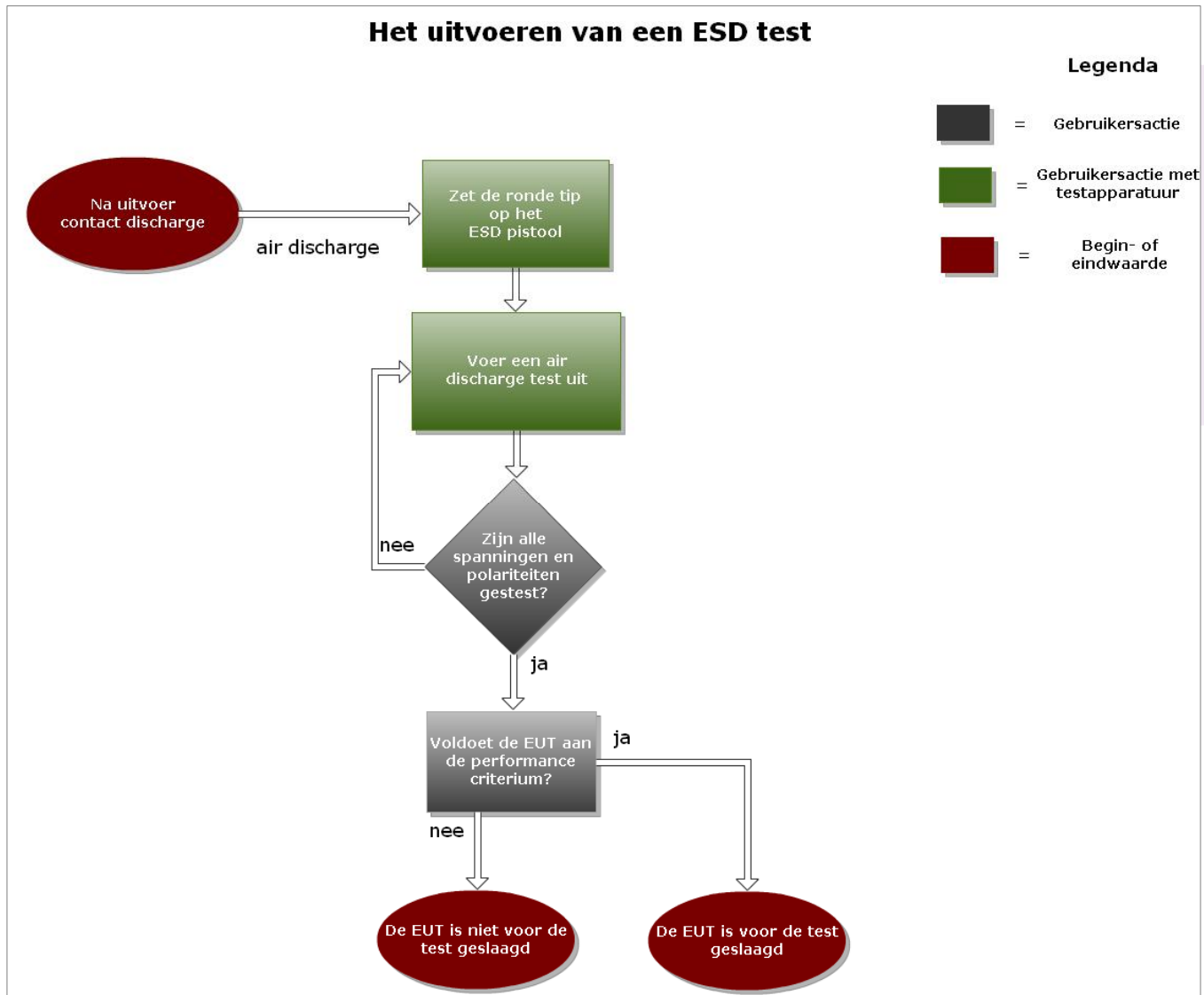
Figuur 10: Het laatste deel van de ESD test met het air discharge testonderdeel.
