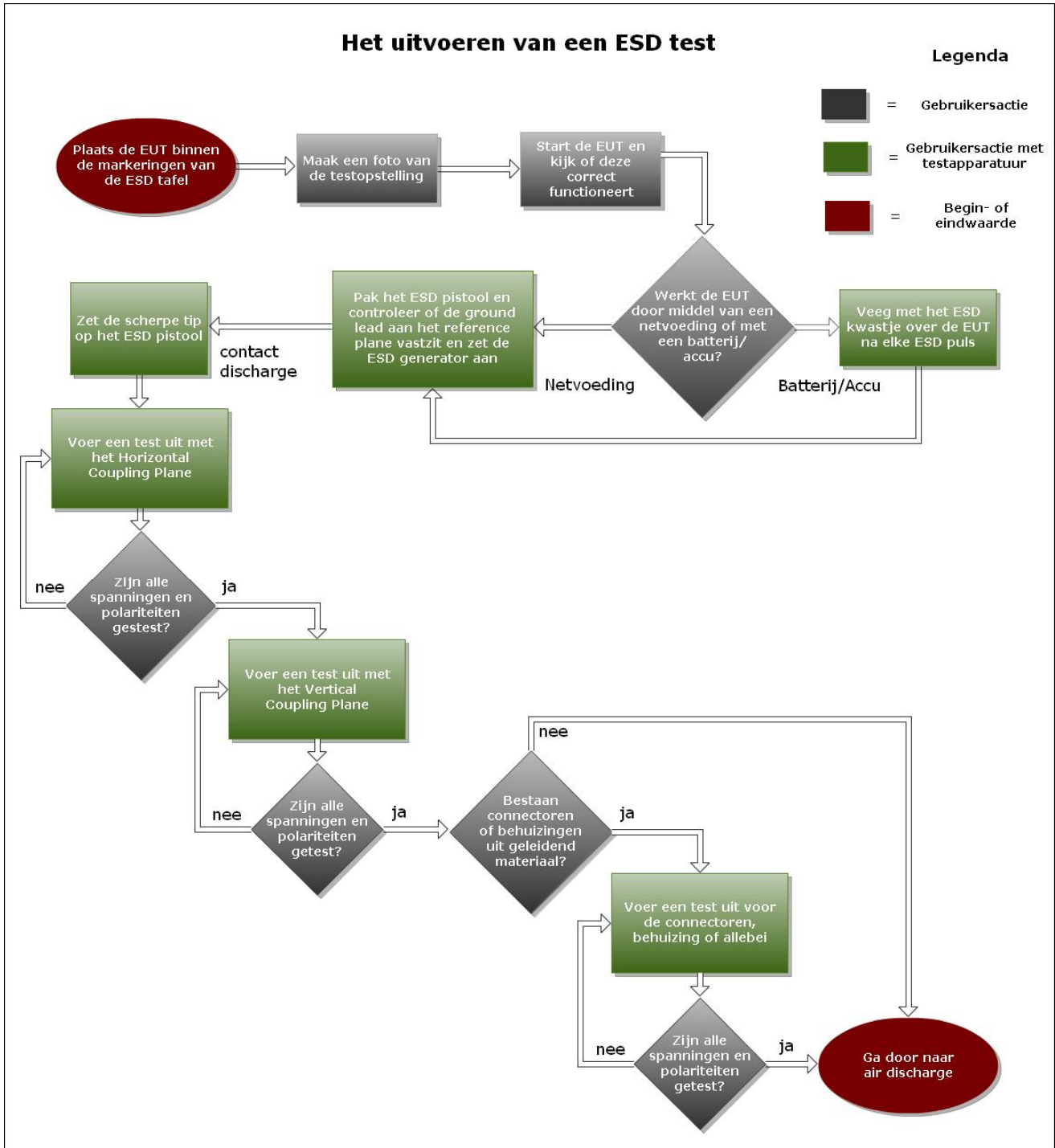
Figuur 9: De start van de ESD test met het contact discharge testonderdeel.
